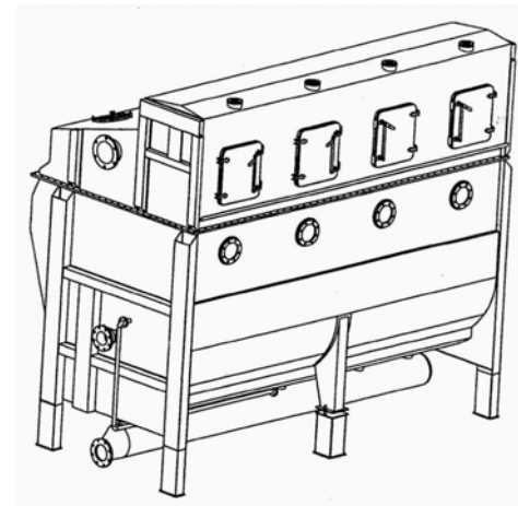
设计3立体图
